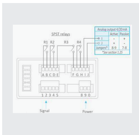
Esquemático Relé ECR 4
