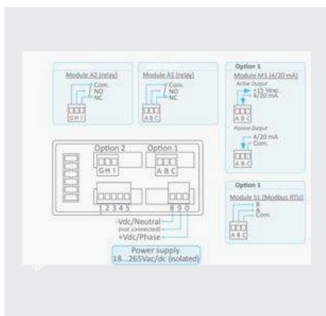
Relé ECR 2 esquemático
