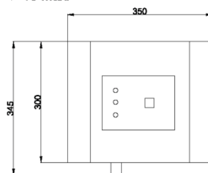
GPS-10 Maxi
